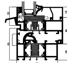
Querschnitt durch das Fenster MB-70 HI
