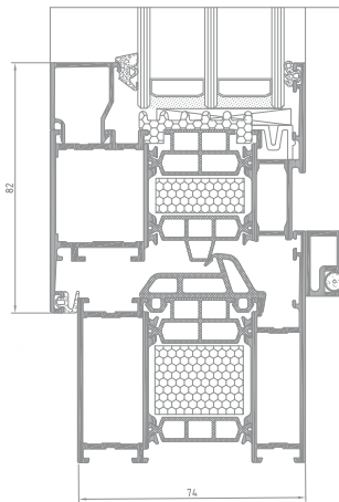
Querschnitt von SP i+, mit Flyscreen verbunden
