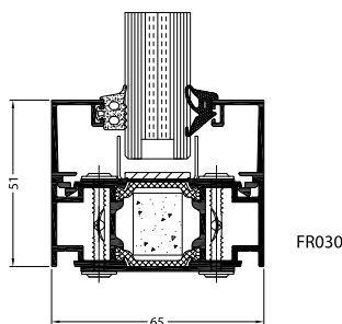
przekrój przez skrzydło FR65
