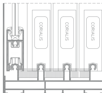
Ecoslide, Querschnitt eines 4-bahnigen Blendrahmens
