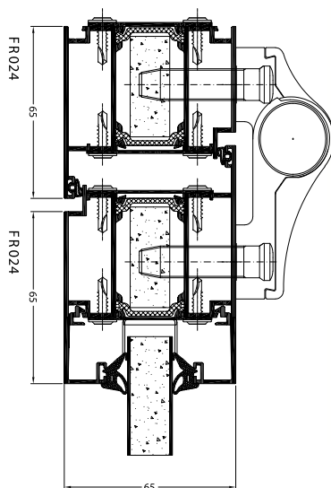
przekrój przez drzwi FR65
