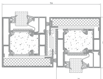
Querschnitt eines festen und beweglichen Flügels im AF-Slide-System
