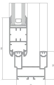
Slide Cold, Querschnitt eines 2-bahnigen Blendrahmens
