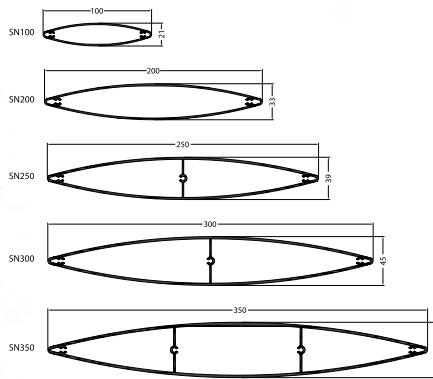
Beispielhafte Außenmasse und Neigungswinkel für Sonnenlamellen des Systems SUN PROTECT
