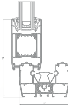
Querschnitt durch den Blendrahmen und den Flügel auf einer Innenbahn
