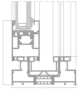
Querschnitt durch eine Tür VG PLUS
