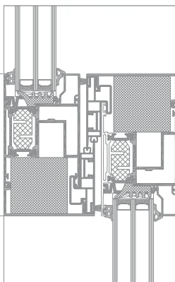
Querschnitt durch eine Flügel-Flügel-Verbindung
