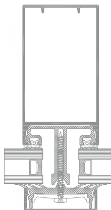
Unterschiedliche Leisten für Innen- und Außenbereich erhältlich
