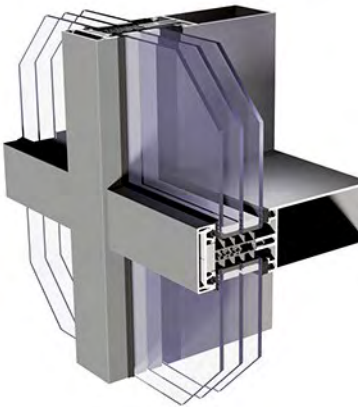
Querschnitt durch den Pfosten MC Passive
