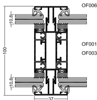
Querschnitt durch eine Tür OFFICE
