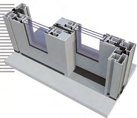
Querschnitt durch Rahmen und Flügel ULTRAGLIDE - Option mit Flachschwelle
