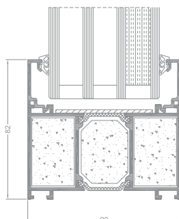
Querschnitt durch den Flügel fix FR90
