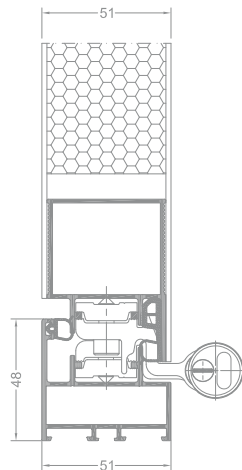
Querschnitt durch eine Paneeltür - Scharnierseite
