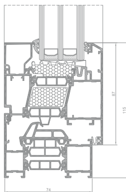
Querschnitt durch ein Fenster SP OUT i+
