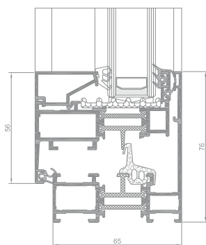
Querschnitt durch ein Fenster IP SU i
