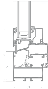
Querschnitt durch ein Fenster
