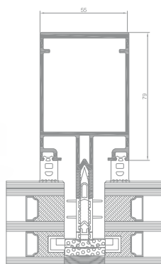
Querschnitt durch den Pfosten MC GLASS
