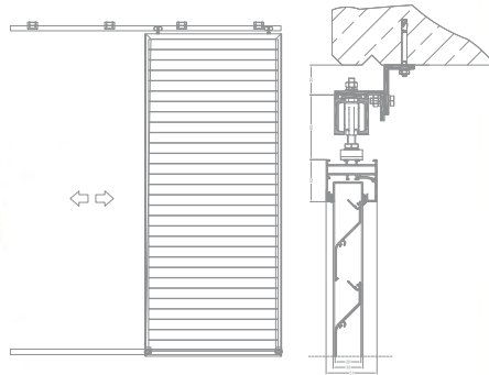
Beispielhafte Außenmasse und Neigungswinkel für Sonnenlamellen des Systems SUN PROTECT
