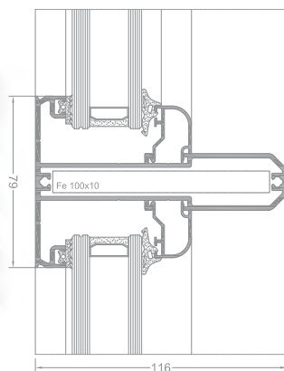
Verglasungsoption mit einer Leiste
