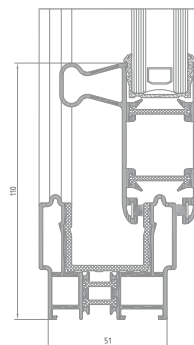
Querschnitt durch eine Tür SL+
