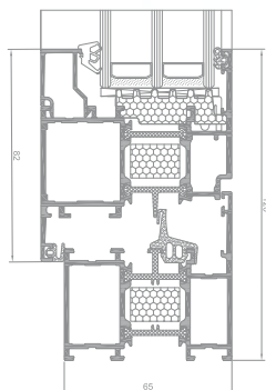
Querschnitt durch ein Fenster IP i+
