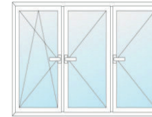
Dreh-Kipp/Dreh/ Dreh Fenster-Tür mit Pfosten ohne Stulp - DK/D/D
