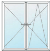
Dreh/Dreh-Kipp Fenster-Tür mit Pfo- sten ohne Stulp - D/DK
