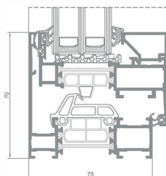
Querschnitt durch ein Fenster SP SU i
