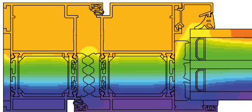
Verteilung der Isothermen in der Tür MB-86N SI+
