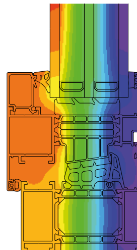
Verteilung der Isothermen im Fenster MB-86N SI
